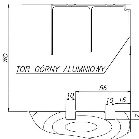
Rys. 4 SYS AL. 20 „AGAT”, „ONYX” „SYS AL. 25 „AGAT II” ORAZ SYS AL 31 “AURORA”
