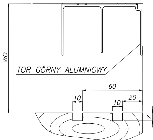
Rys. 3 SYS AL. 20 „LAZURYT”, „ARTDECO” ORAZ SYS AL. 25 „LAZURYT II”
