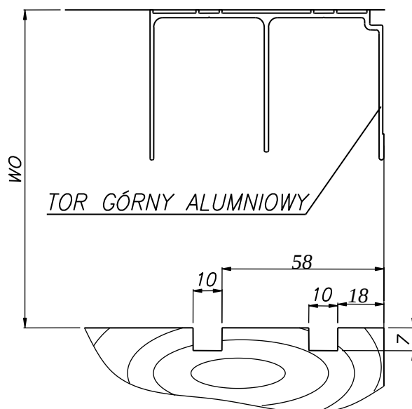
Rys. 5 SYS AL. 25 „SZAFIR”
